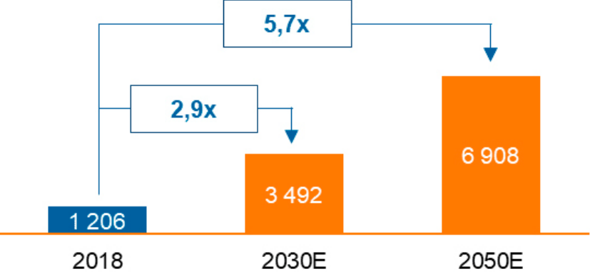
Maaanlaajuiset aurinko- ja tuulivoiman tuotantokustannukset LCOE-menetelmällä laskettuna ($/MWh, 2019 hinnoin) 2)
